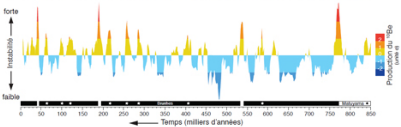
Episodes de surproduction du nucléide cosmogénique Béryllium-10 pendant des phases d'instabilités du champ magnétique terrestre
